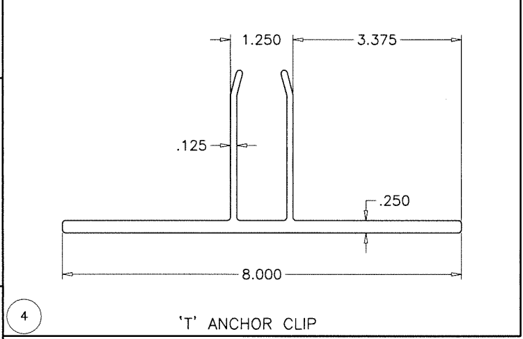
4 'T' ANCHOR CLIP
